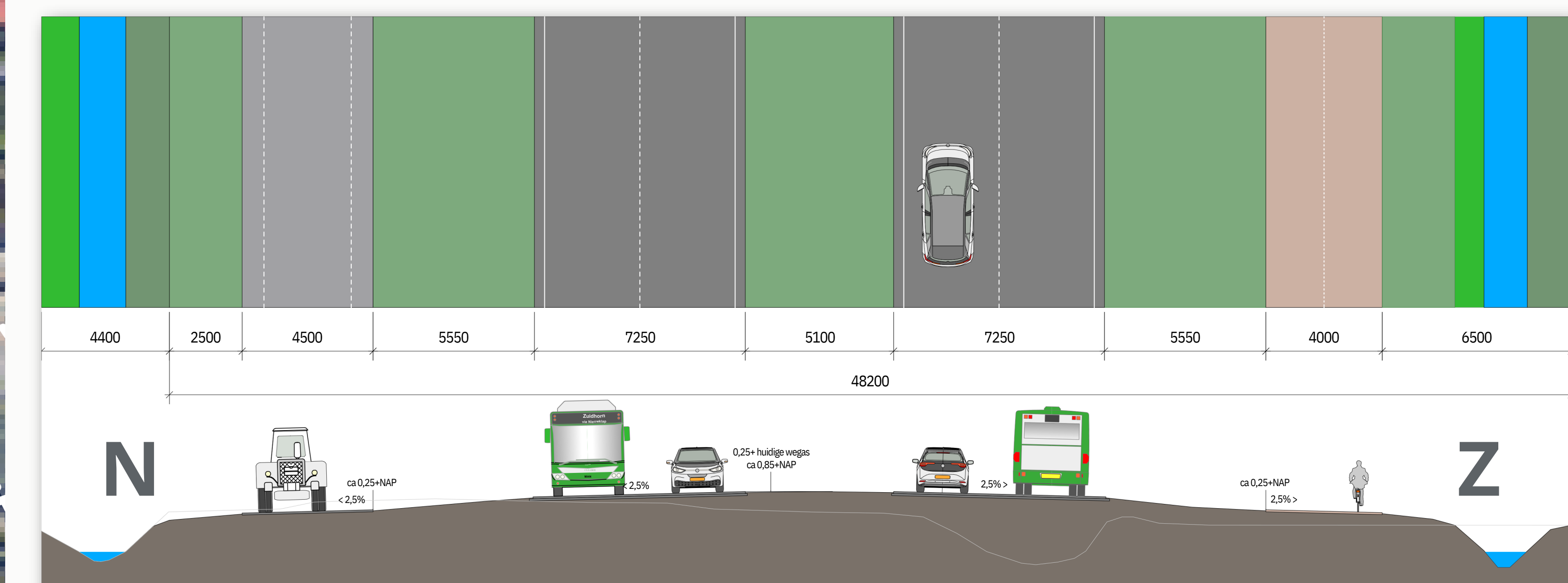
Wegprofiel nieuwe situatie
