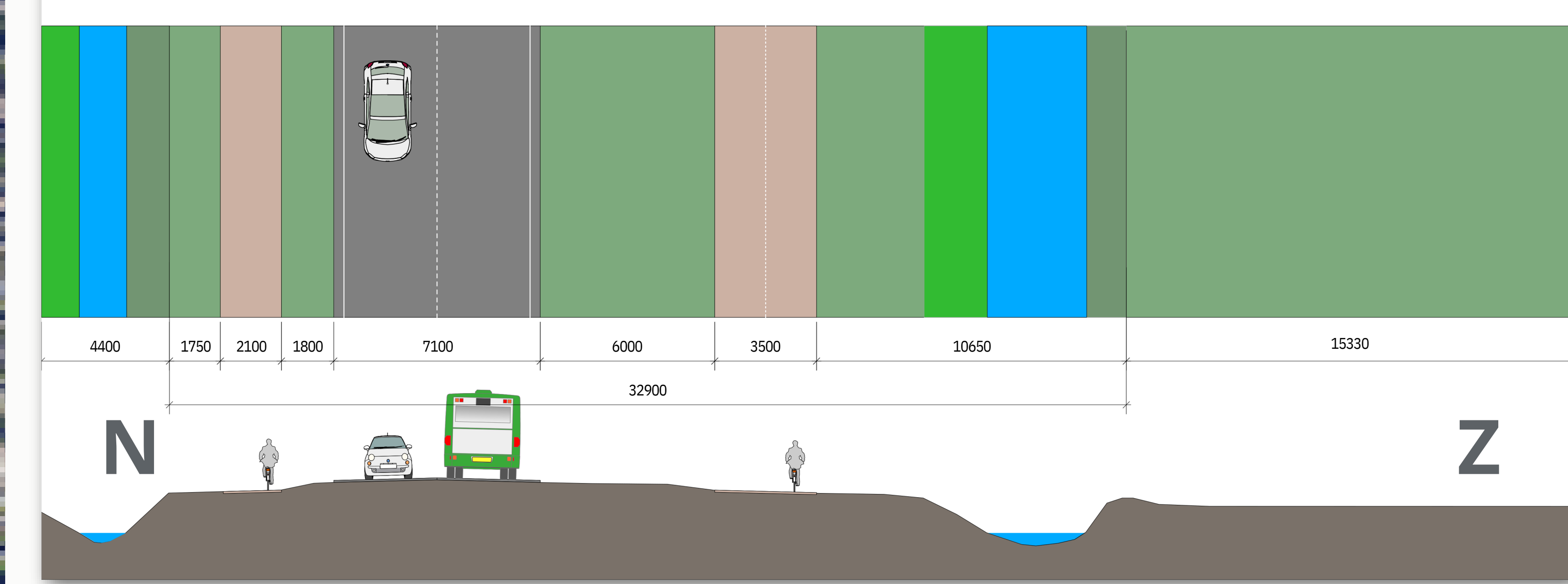
Wegprofiel huidige situatie
